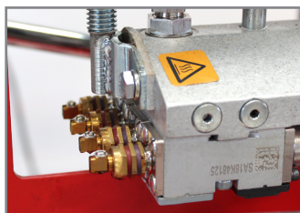
SISTEMA CHIUSURA COLLA A CALDO GLUE CLOSER SYSTEM
