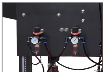
PARTICOLARE PNEUMATICO PNEUMATIC DETAIL
