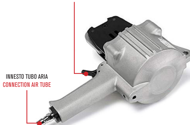
PULSANTE DI AZIONAMENTO BUTTON SWITCH
