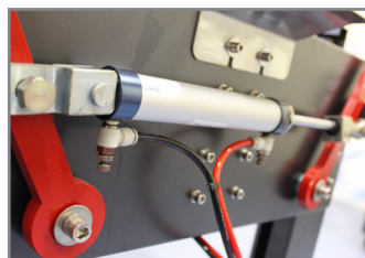
SISTEMA PNEUMATICO PER CHIUSURA FALDE PNEUMATIC SYSTEM FOR FLAPS CLOSURE
